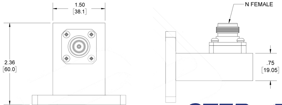
WR137 CPRG FLANGE
