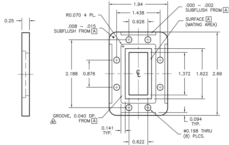
WR137 CPRG FLANGE
