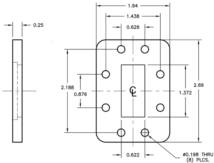
WR137 CPRF FLANGE
