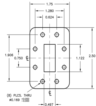
CPRF FLANGE (R)
