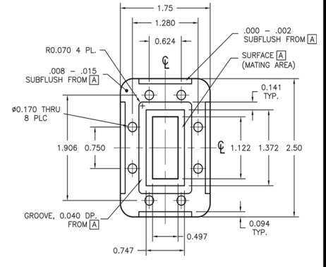
CPRG FLANGE (G)
